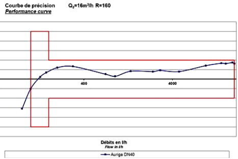
Мал. 2 Графіки залежності відносної похибки лічильників від об'ємної витрати
