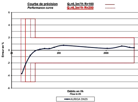
Мал. 2 Графіки залежності відносної похибки лічильників від об'ємної витрати
